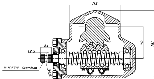
SEC:B-B
