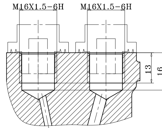
Sec A-A Scale(2:1)
