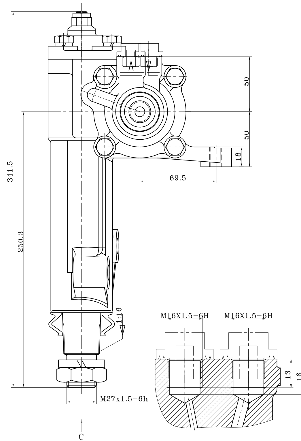
Sec A-A Scale(2:1)
